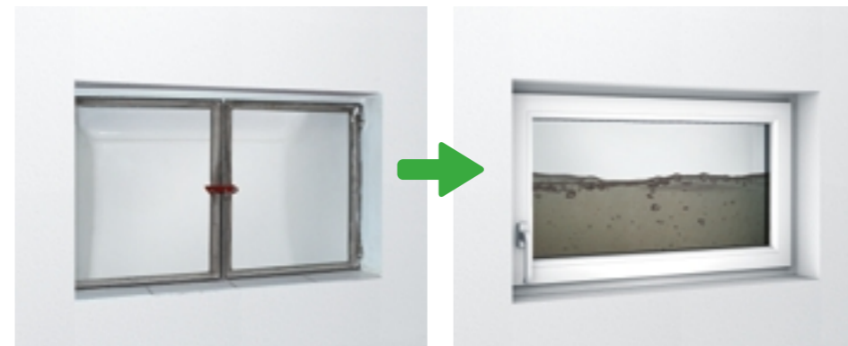
Umbau Stahlfenster mit Glas auf hochwertiges, wasserdichtes Dreh-Kipp-Fenster
